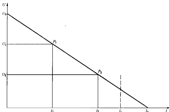
图 2 电流发生器的负载特性
